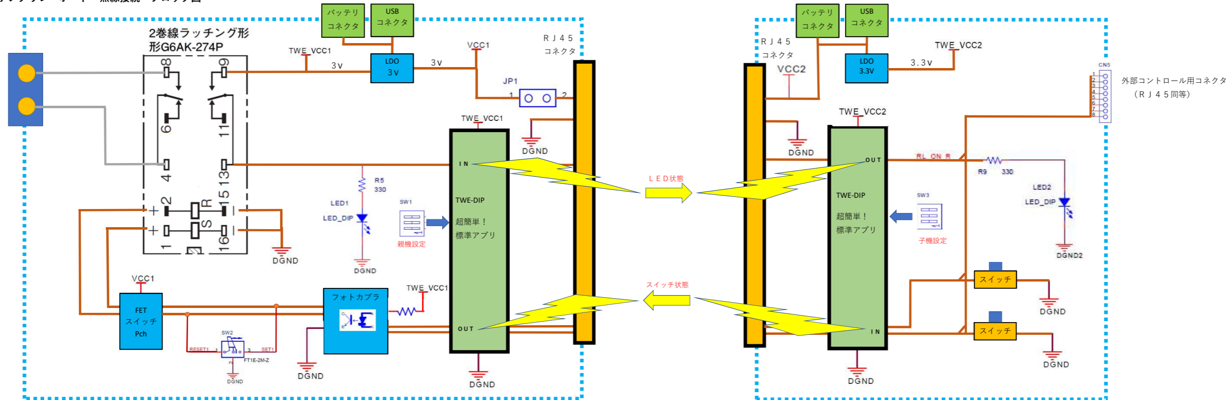
ラッチングリレーボード 無線接続 ブロック図
