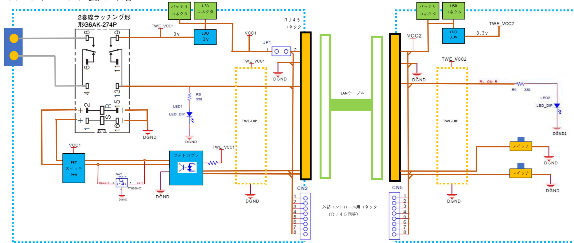
ラッチングリレーボード LANケーブル接続 ブロック図
